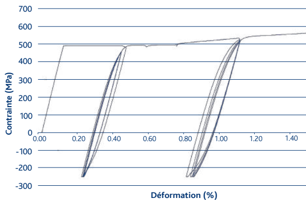
Diagramme contrainte-déformation. Simulation sismique par essai cyclique selon les prescriptions ISO 15835-1
