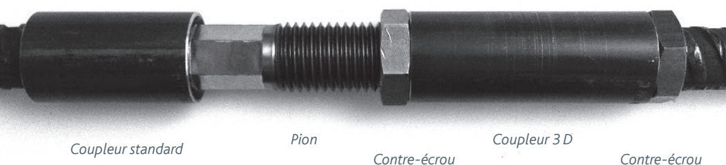
Contre-écrou
