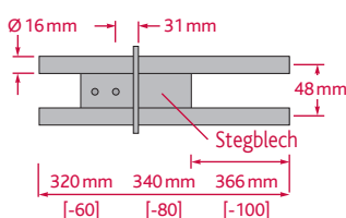
DSDS 30 – Doppelschubdorn
