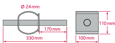
ADH 24 – Hochlastdorn
