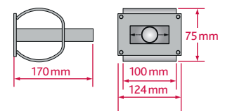
AHQ 18 – Hochlast-Stahlhülse mit Querweg ( \pm 12 mm)
