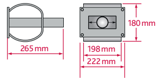
AHQ 42 – Hochlast-Stahlhülse mit Querweg ( \pm 23 mm)
