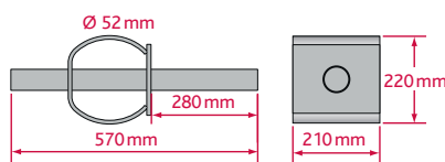
ADH 52 – Hochlastdorn
