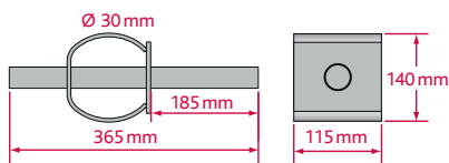
ADH 30 – Hochlastdorn
