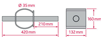
ADH 35 – Hochlastdorn
