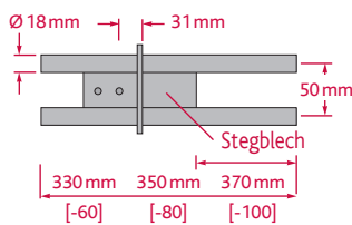
DSDS 50 – Doppelschubdorn
