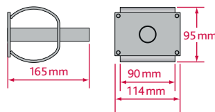
AHS 22 – Hochlast-Stahlhülse
