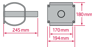
AHS 42 – Hochlast-Stahlhülse
