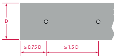
konstruktive Mindestabstände
