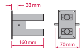
DSDSQ 50 – Stahlhülse mit Querweg ( \pm 12 mm)
