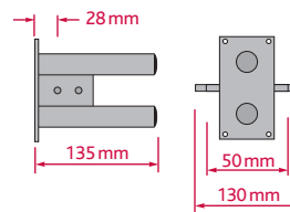
DSDS 50 – Stahlhülse
