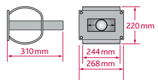
AHQ 52 – Hochlast-Stahlhülse mit Querweg ( \pm 19 mm)
