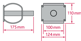
AHS 24 – Hochlast-Stahlhülse
