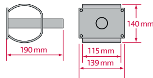
AHS 30 – Hochlast-Stahlhülse
