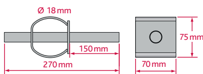
ADH 18 – Hochlastdorn
