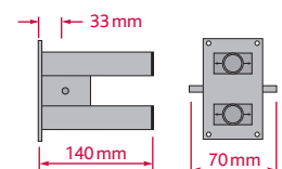
DSDSQ 30 – Stahlhülse mit Querweg (±13 mm)
