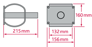
AHS 35 – Hochlast-Stahlhülse
