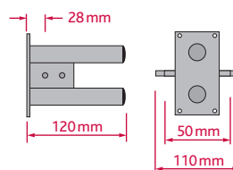
DSDS 30 – Stahlhülse
