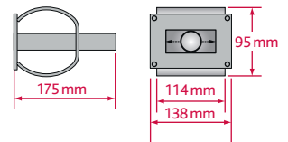
AHQ 22 – Hochlast-Stahlhülse mit Querweg ( \pm 10 mm)
