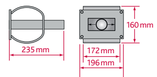
AHQ 35 – Hochlast-Stahlhülse mit Querweg ( \pm 16 mm)
