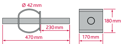
ADH 42 – Hochlastdorn
