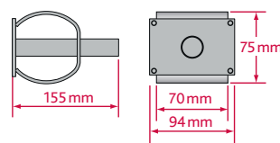
AHS 18 – Hochlast-Stahlhülse
