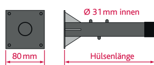
AKH 20 – Kunststoffhülse
