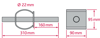
ADH 22 – Hochlastdorn
