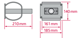
AHQ 30 – Hochlast-Stahlhülse mit Querweg ( \pm 20 mm)
