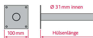
ASH 20 – Stahlhülse
