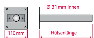
AQH 20 – Stahlhülse mit Querweg (± 20 mm)
