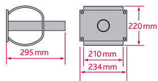
AHS 52 – Hochlast-Stahlhülse
