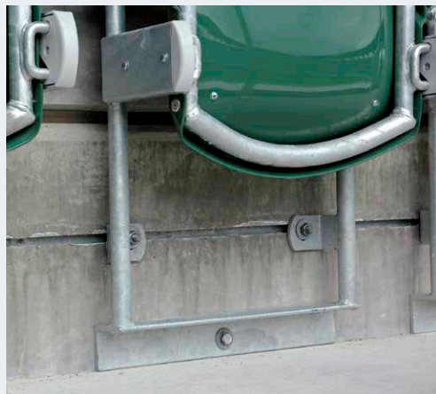
Les sièges ont nécessité 18'000 vis à béton MULTI-MONTI et 36'000 boulons d'ancrage.
