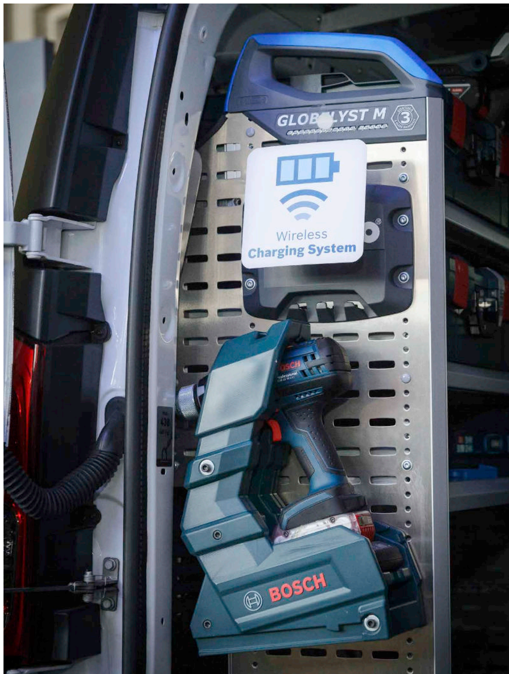
Ce support permet par exemple d'y accrocher l'outil pendant vos déplacements. Il se recharge pendant le trajet.
